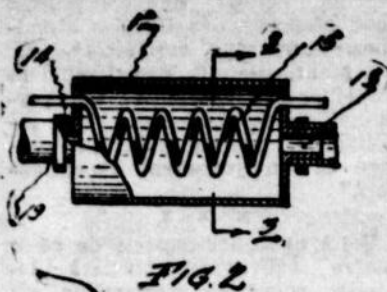
Une coupe du serpentin où se réchauffe l'essence.
