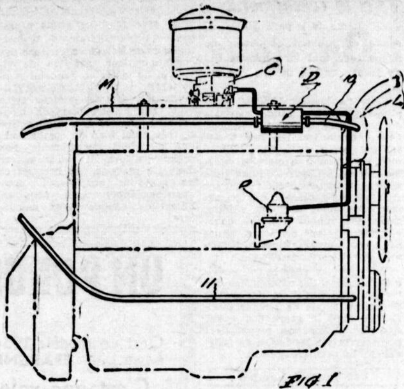
Voici comment s'installe sur le moteur (à droite) l'appareil de M. Jean-Marc Tremblay.
